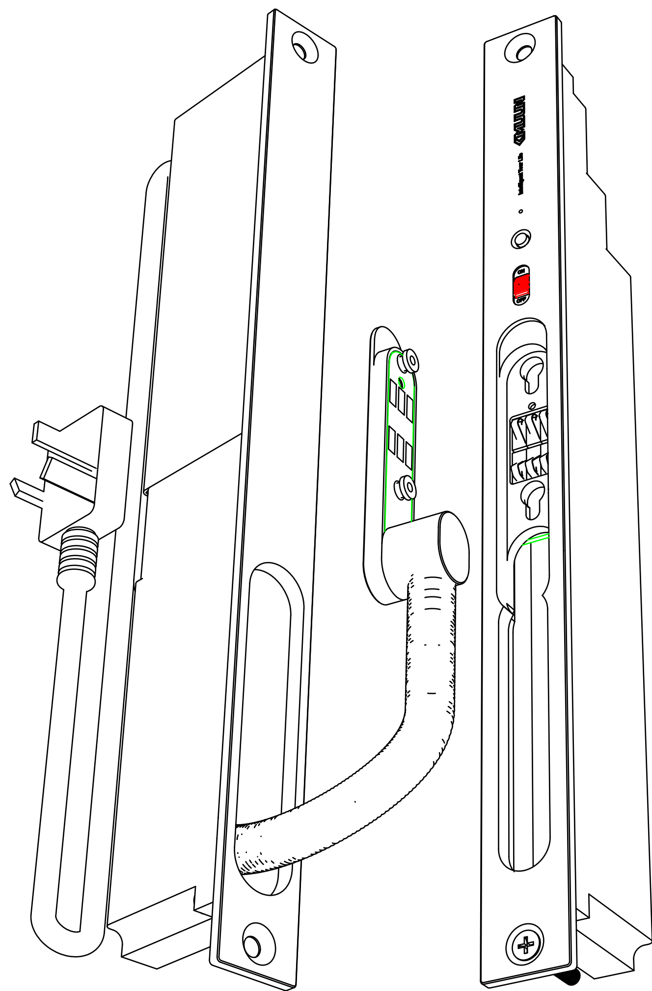
安装于门框
