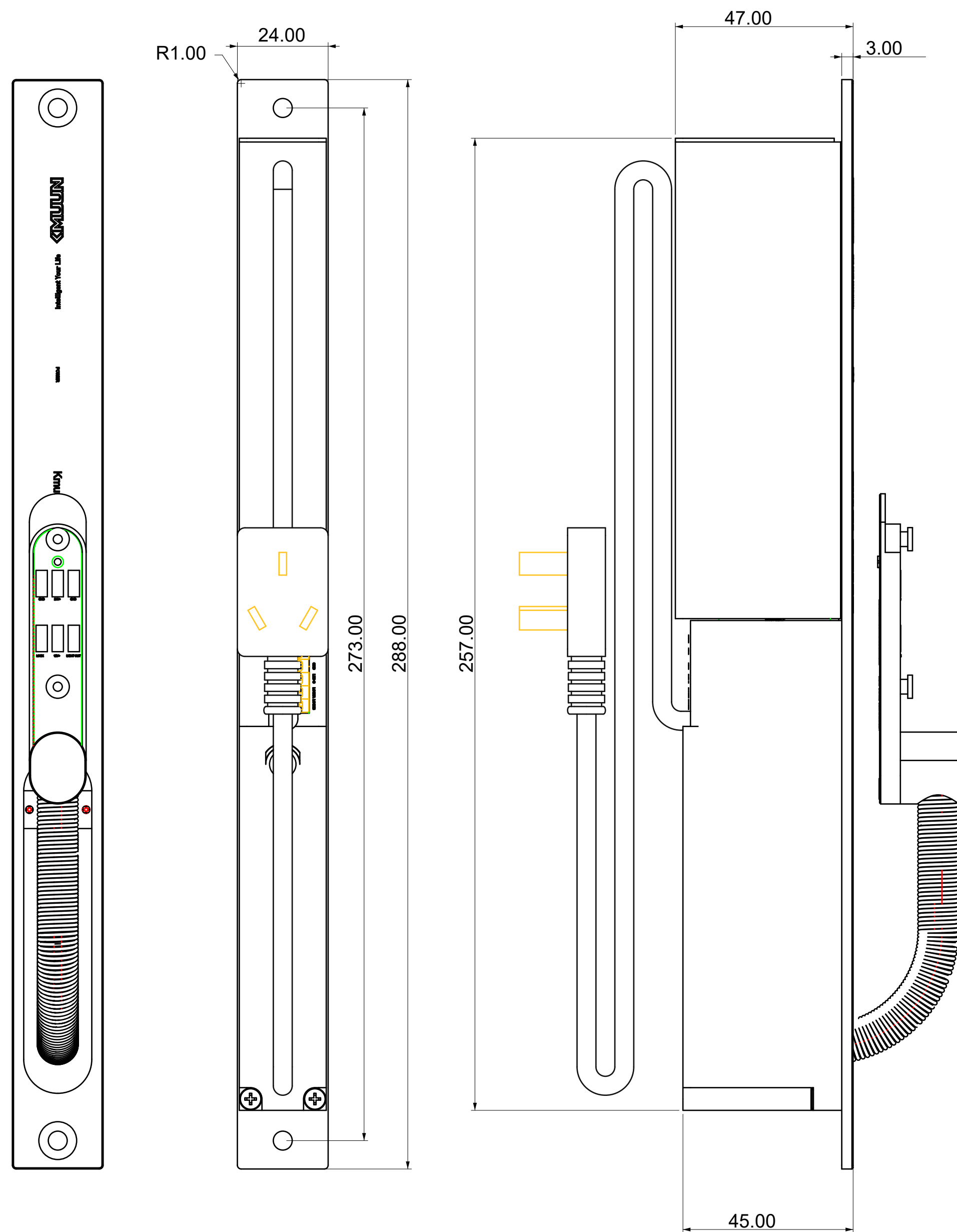
安装于门框
