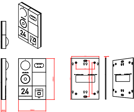
室外机-横装
