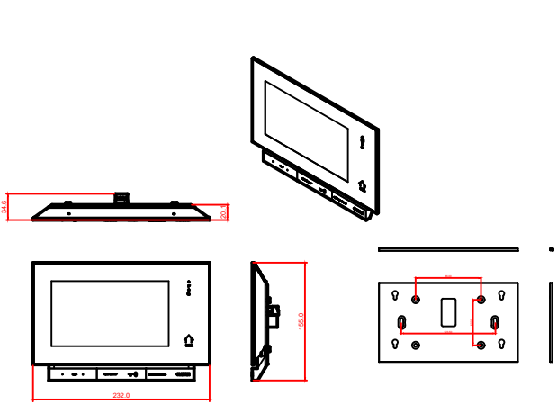
室内主机
