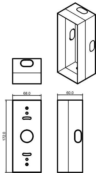
外机预埋盒
