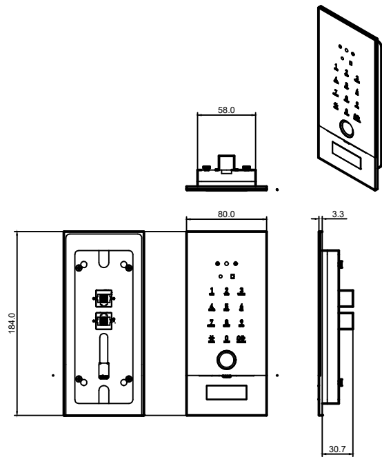
外机主体
