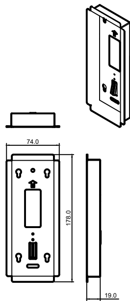
外机安装底盒
