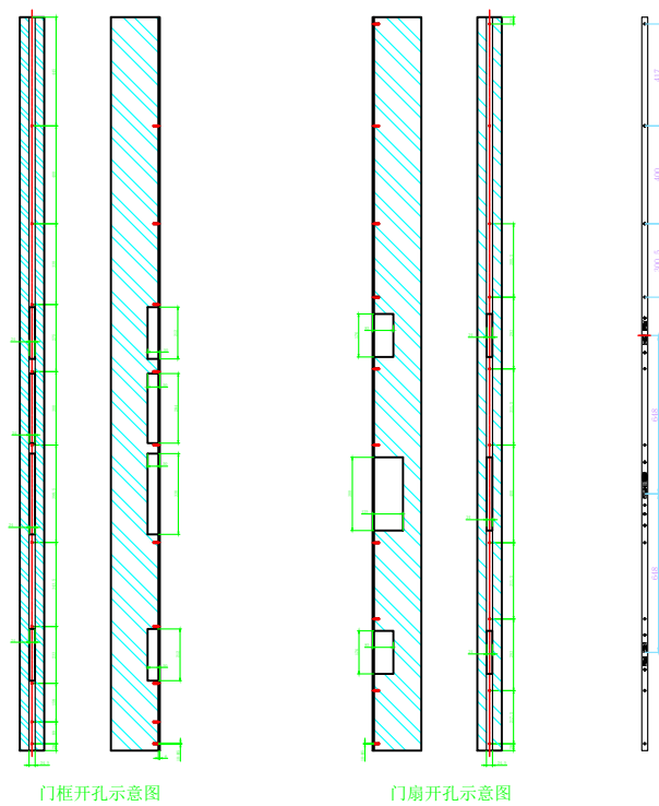
门扇开孔示意图
